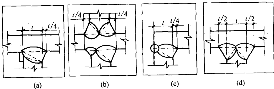
图 5.2.5 焊脚尺寸
